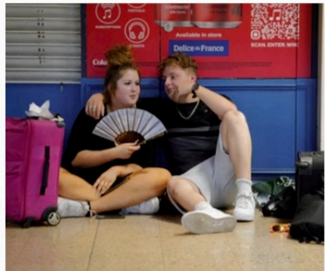
TEMPERATURA No aeroporto de Heathrow foram registrados 40,2°C
